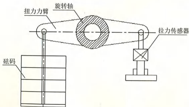
图5 扭矩校准安装示意图
