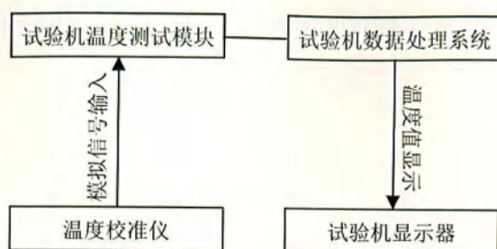
图4 温度校准仪校准原理图
