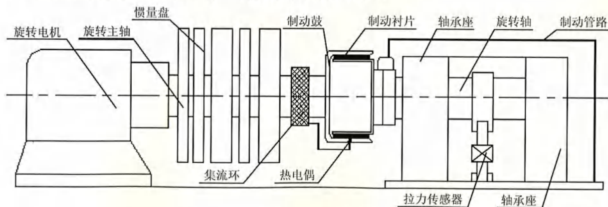
图1 商用车制动器惯性试验台结构示意图
